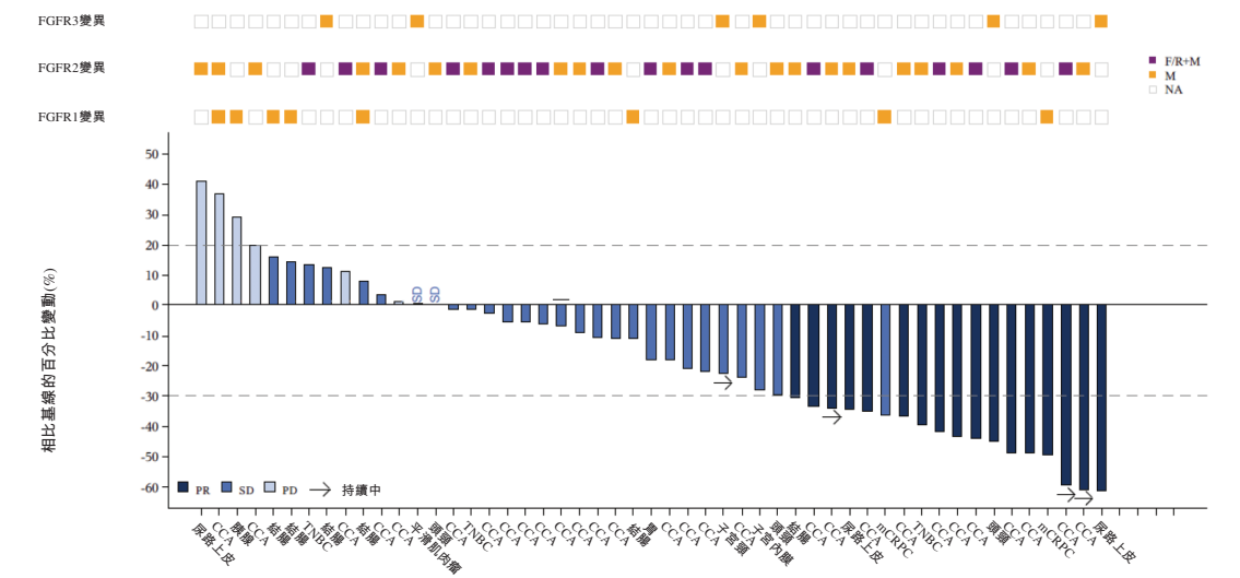
具有FGFR1/2/3變異的泛腫瘤瀑布圖(N=51)
