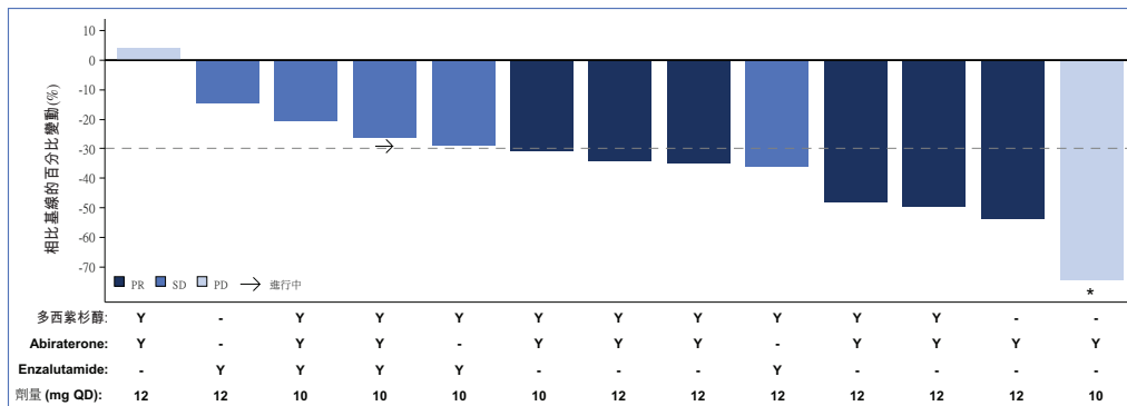
mCRPC患者的瀑布圖(N=13)
