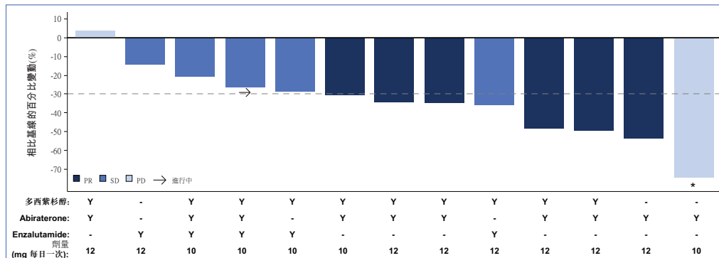
mCRPC患者的瀑布圖(N=13)
